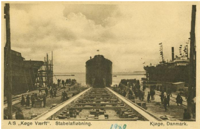
A.S. „Køge Værft“, Stabelafløbning. 1920 Kjøge, Danmark. Stabelafløbning i 1920 af NERMA , det første stålskib bygget på Køge Værft. Skibet blev leveret til rederiet J.L. Lauritzen , Esbjerg i 1921. Foto: Køge Byhistoriske Arkiv.
